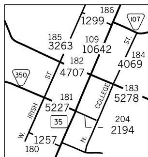
(INSET) 30A
